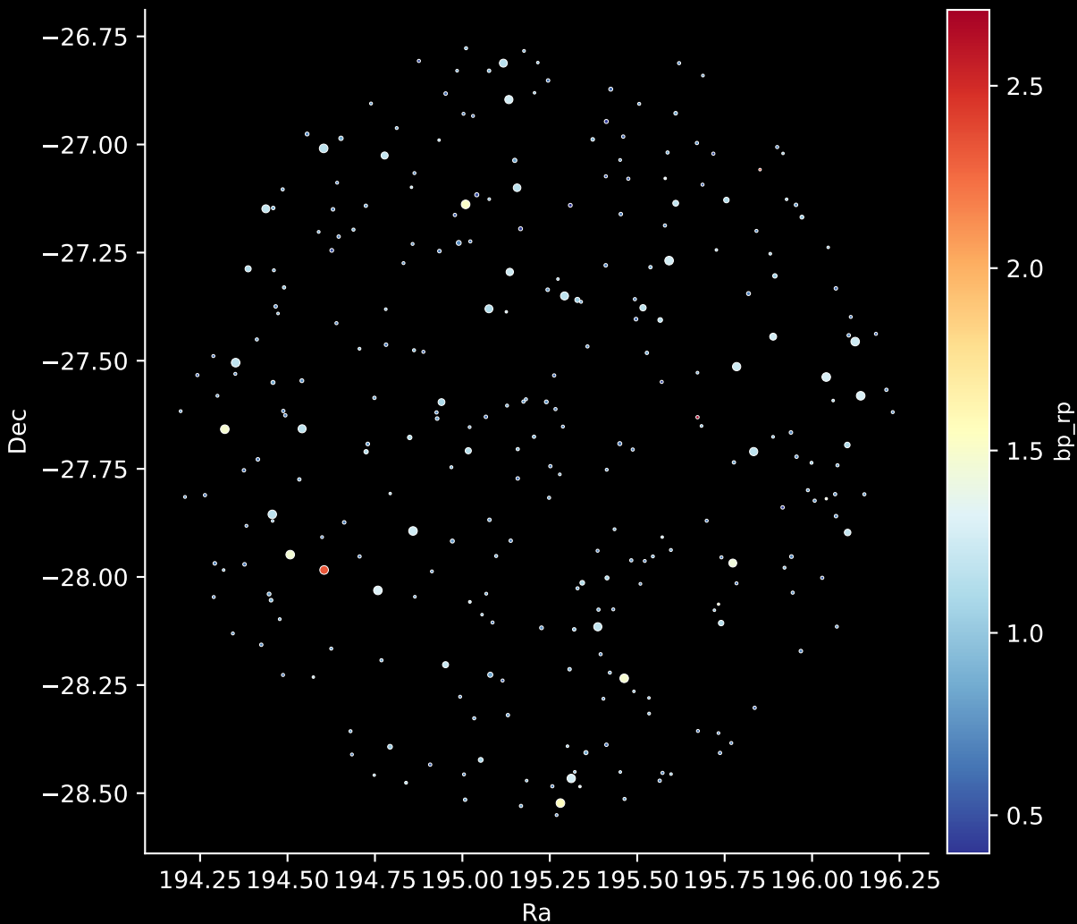
GALAH DR4 Field: [2397] Stars: 289
