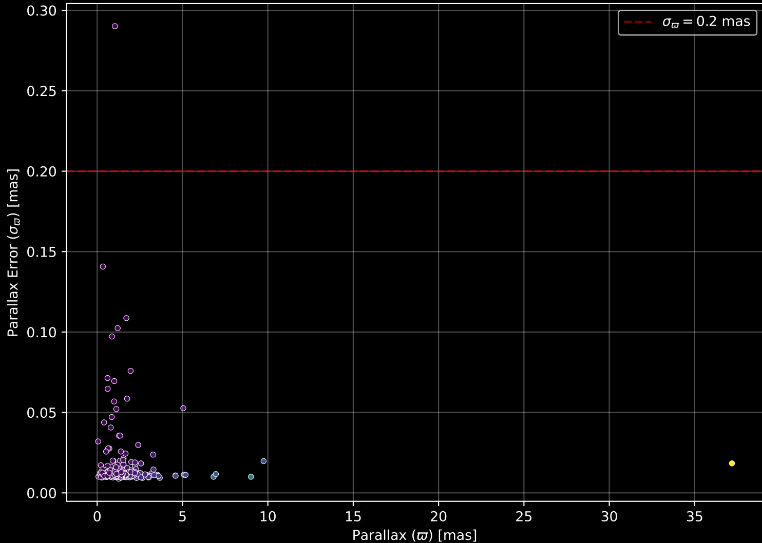
GALAH DR4 Field: [2397] Parallax Quality (n= 289)
